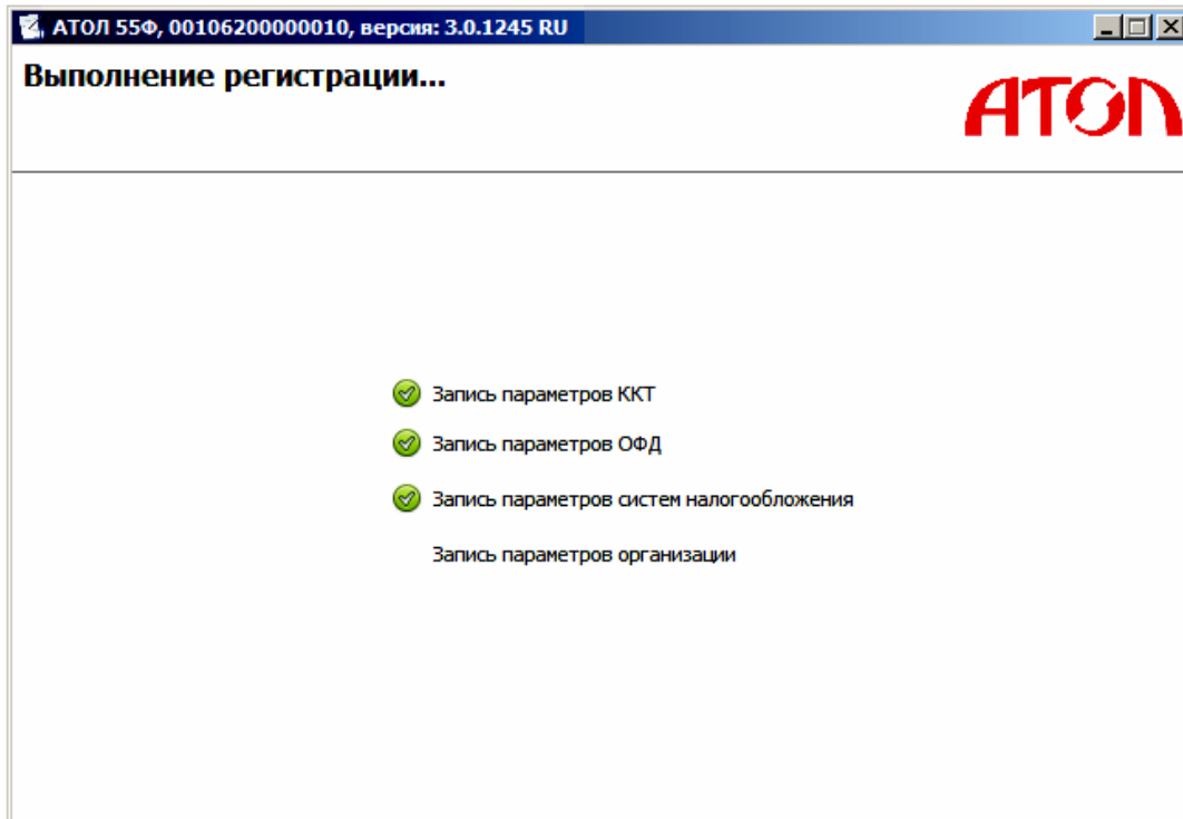
Рисунок 13. Окно информации
